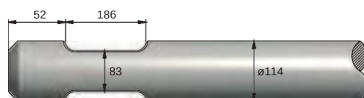
FIGURE 151 ITALDEM GK 1350
